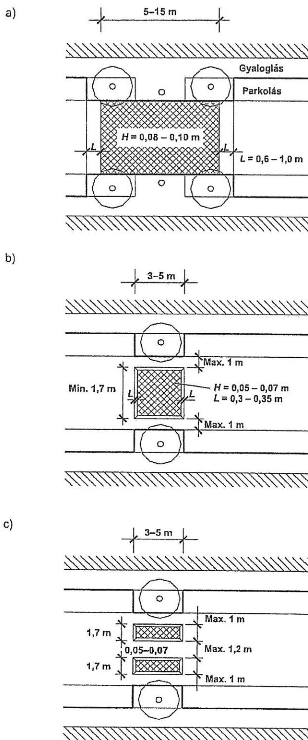
16. ábra – Szintemelések főbb méretei
