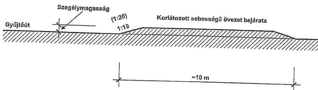
14. ábra – Pályaszintemelések főbb méretei
