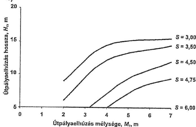
20. ábra – Lakott területen, 50 km/óránál kisebb tervezési sebesség esetén alkalmazható sávelhúzások méretei, kialakítása
