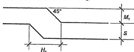
20. ábra – Lakott területen, 50 km/óránál kisebb tervezési sebesség esetén alkalmazható sávelhúzások méretei, kialakítása
