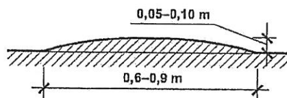
18. ábra – A sebességcsökkentő küszöb főbb méretei
