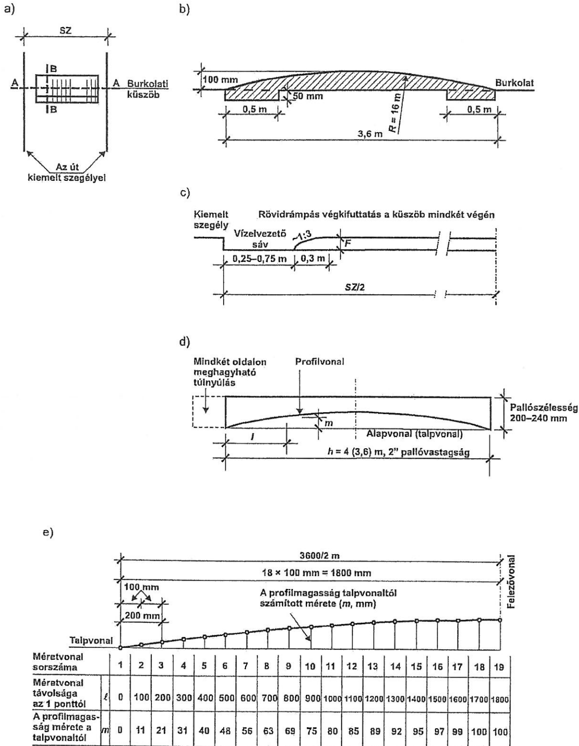
15. ábra – Íves keresztmetszetű pályaszintemelés mintaszelvénye (arányrajz) és ellenőrző sablonjának méretei. (A méretek R=16 m sugarú küszöbök kitűzési adatai);
