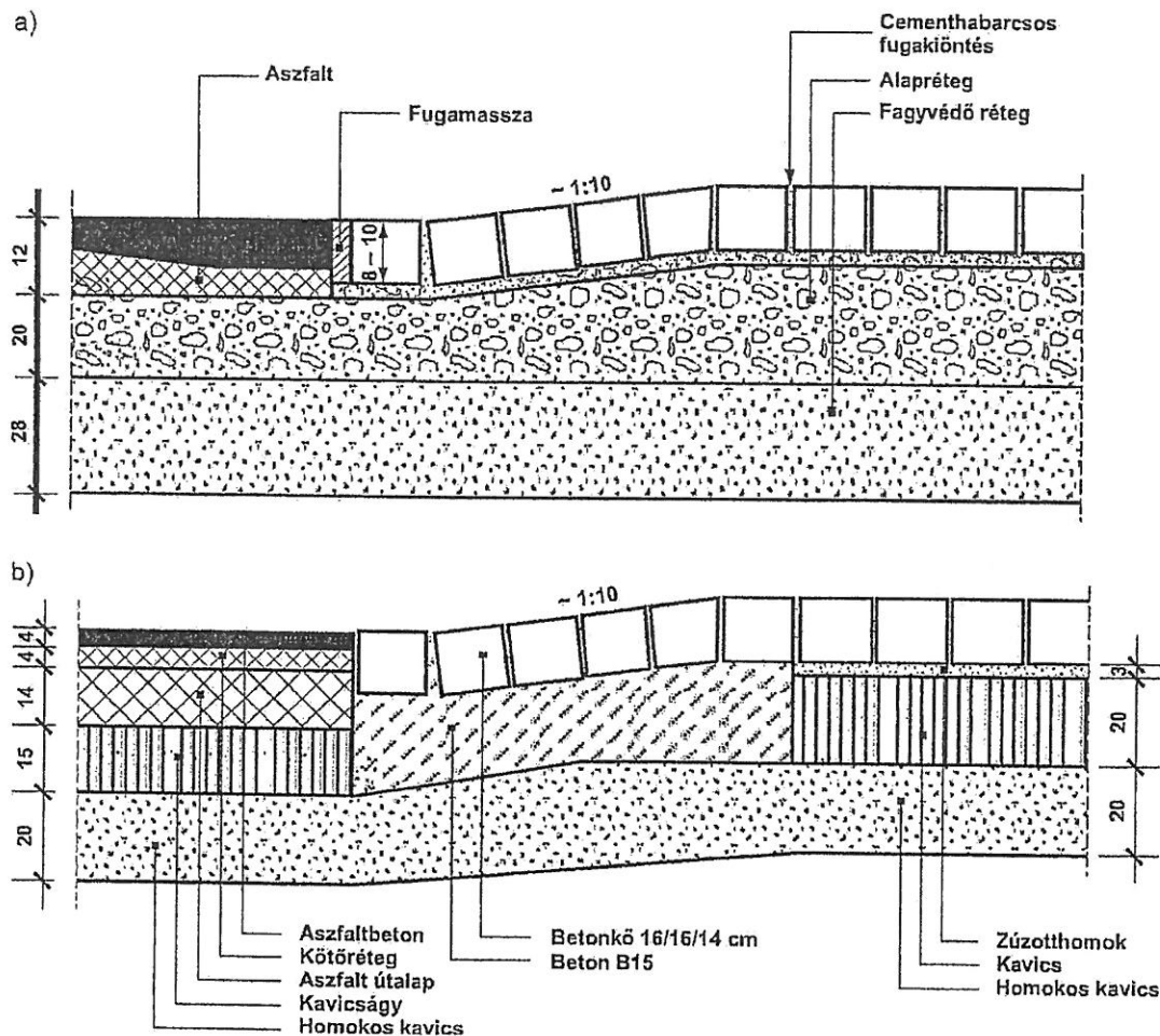
17. ábra – Pályaszintemelés pályaszerkezete (példa)
